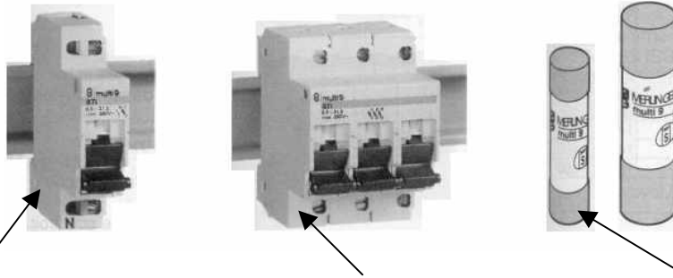
Sectionneur « uni »
